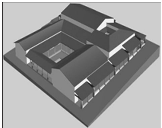
Fig. 14. Modelo 3D da casa das Carvalheiras (Fase I), segundo restituição do arquitecto Rui Silva (laboratório multimédia da UAUM).
