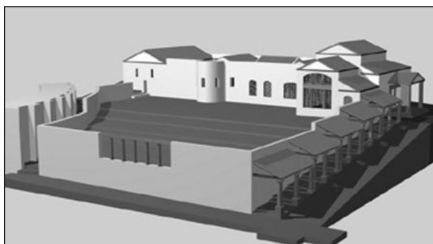
Fig. 8: Modelo 3D da Fase I das termas, segundo proposta da arquitecta Paula Silva (Lab. Multimédia da UAUM).
