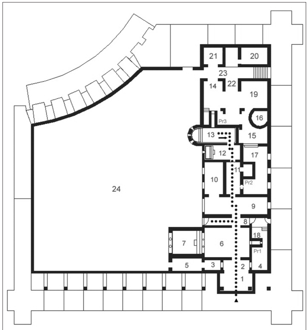
Fig. 7: Planta do edifício das termas do Alto da Cividade na Fase I: 1 e 2: entrada; 3 e 4: cubicular; 5. latrinae; 6. apodyterium; 7. piscina; 8. corredor; 9 e 10. frigidaria; 11 e 12 tepidaria; 13. caldarium; 14 a 23. áreas de serviços; 24. palaestra.
