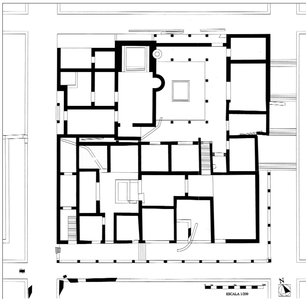
Fig. 15. Planta das Carvalheiras, Fase II.
