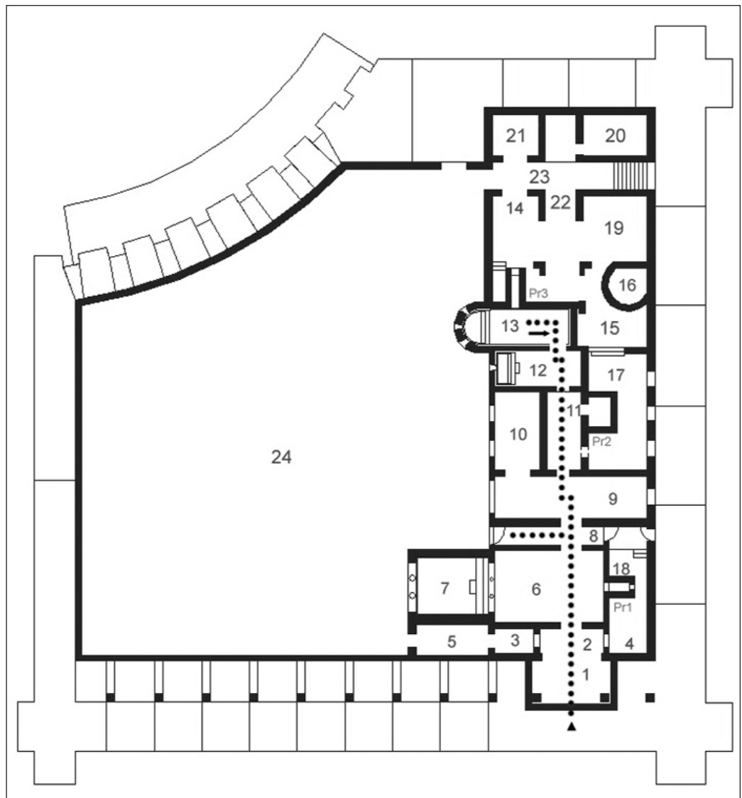
Fig. 7: Planta do edifício das termas do Alto da Cividade na Fase I: 1 e 2: entrada; 3 e 4: cubicalae; 5. latrinae; 6. apodyterium; 7. piscina; 8. corredor; 9 e 10. frigidaria; 11 e 12 tepidaria; 13. caldarium; 14 a 23. áreas de serviços; 24. palaestra.
