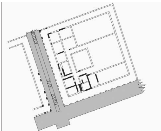
Fig. 12. Planta simplificada das estruturas encontradas no logradouro do edifício do Ex-Albergue Distrital. São visíveis os pórticos, ladeando as construções de ambos os lados da rua, sob a qual corre a cloaca.
